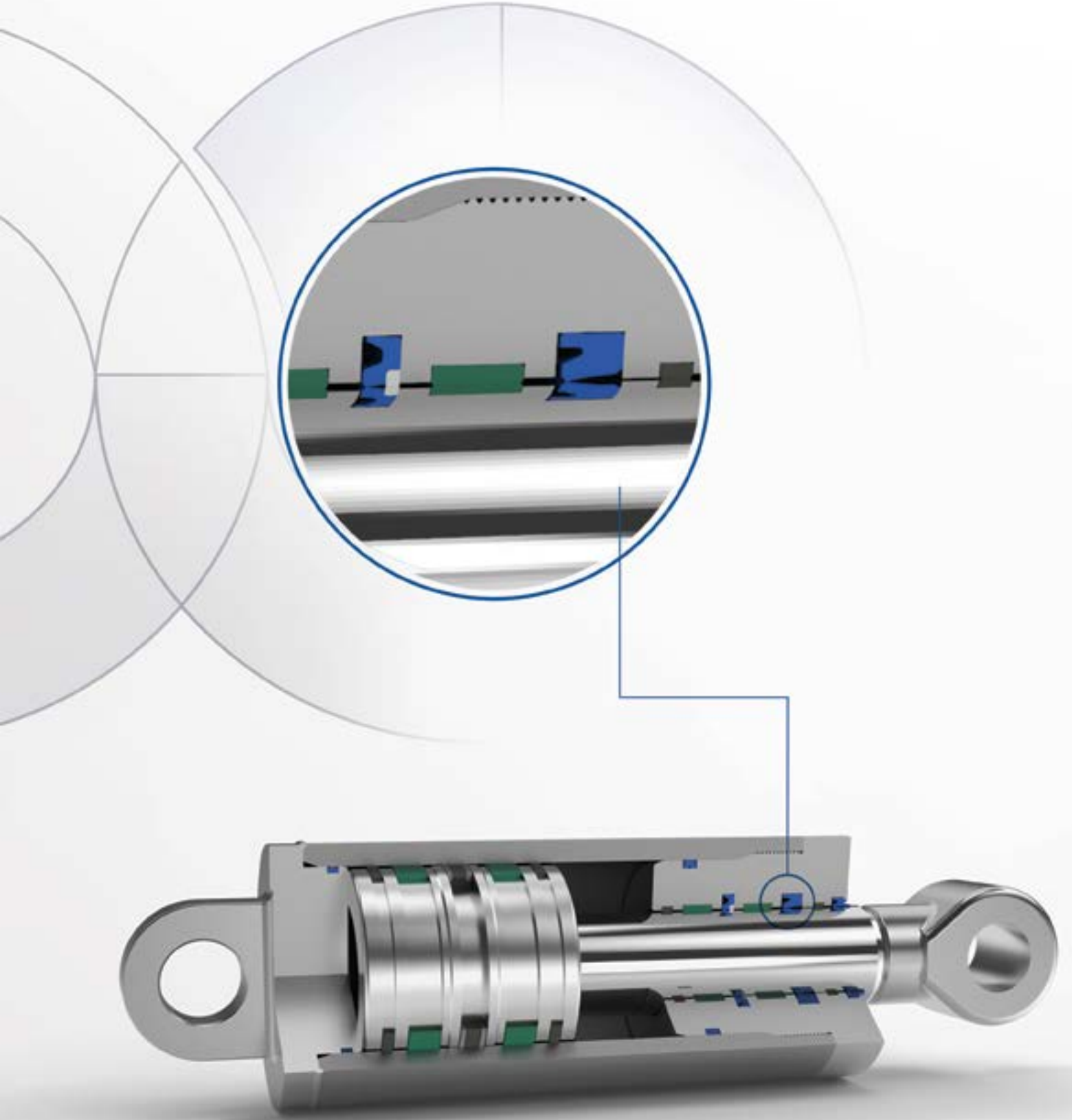
Hidrolik Boğaz Sızdırmazlık Elemanları
