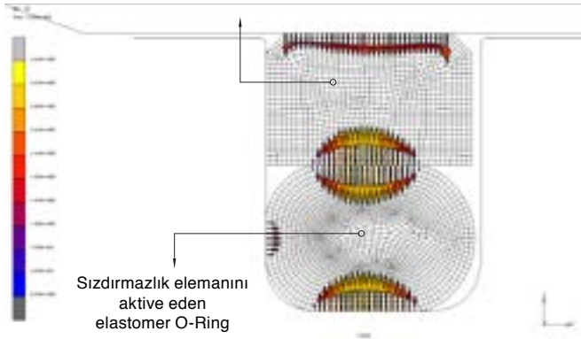
K17 SEA basınçsız durumda temas gerilimi
