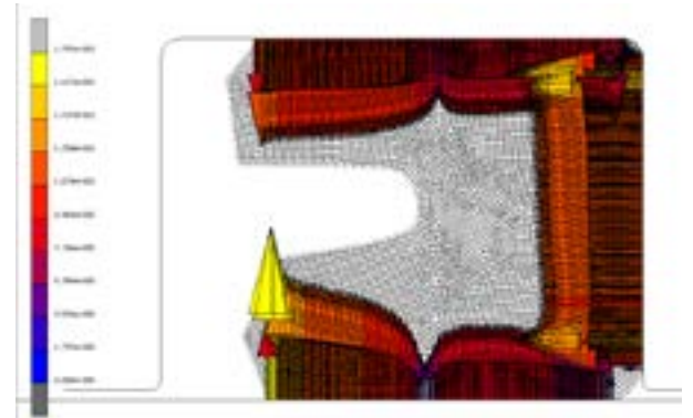
XT200®-050/1 200 bar basınç altında SEA analizi S akma boşluğu: 0.4 mm
